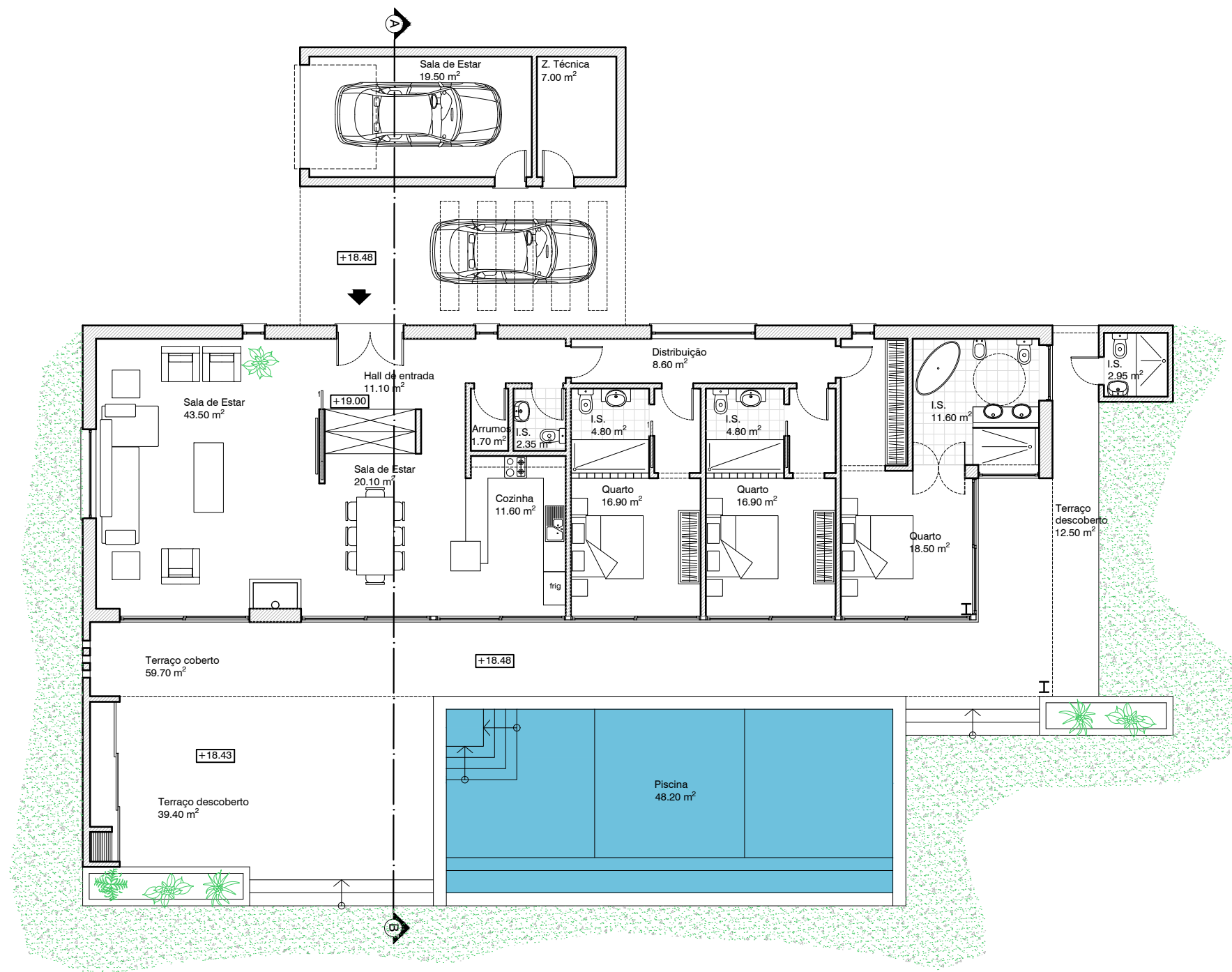
Planta do R/Chão +17.97
