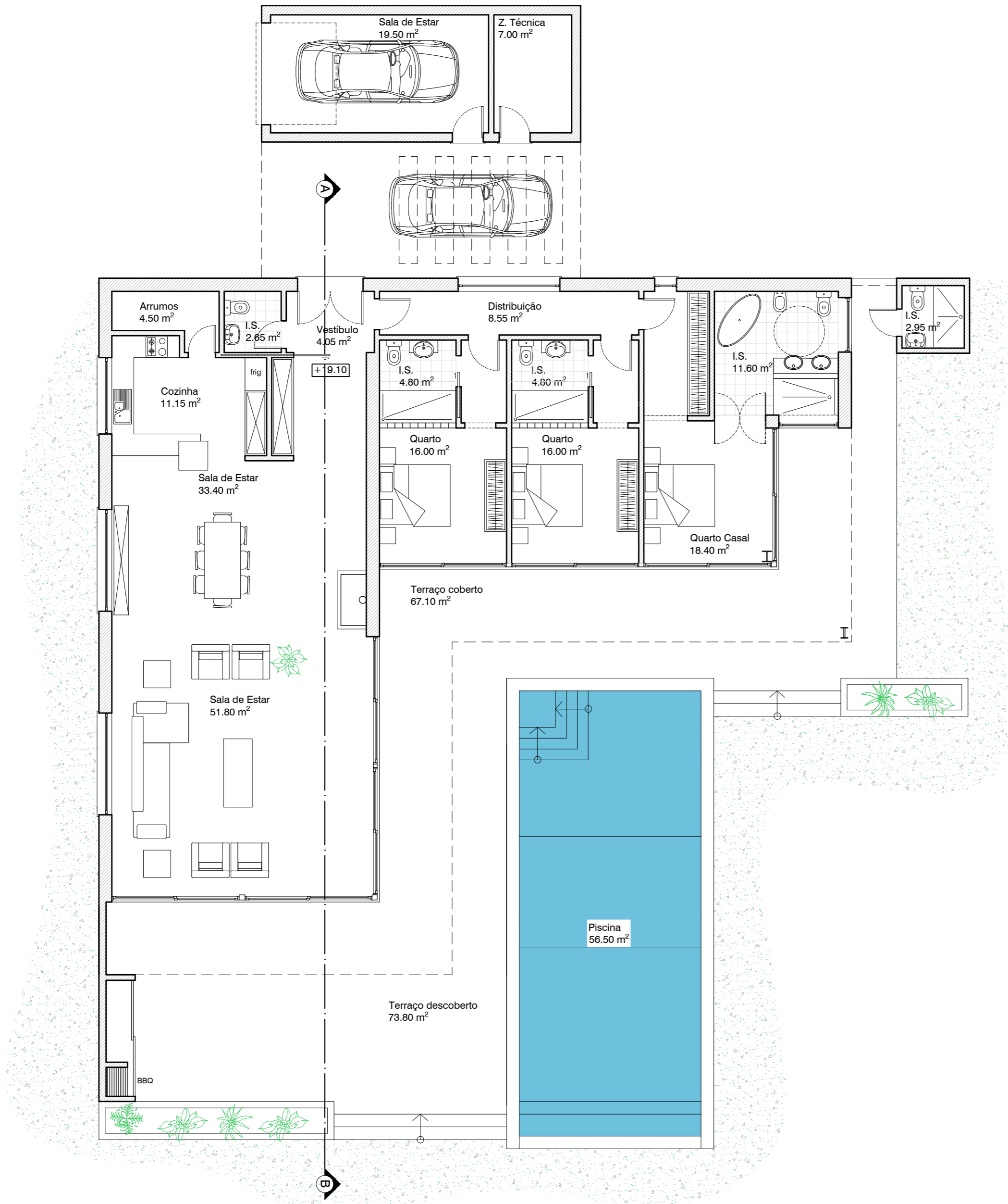
Planta do R/Chão
